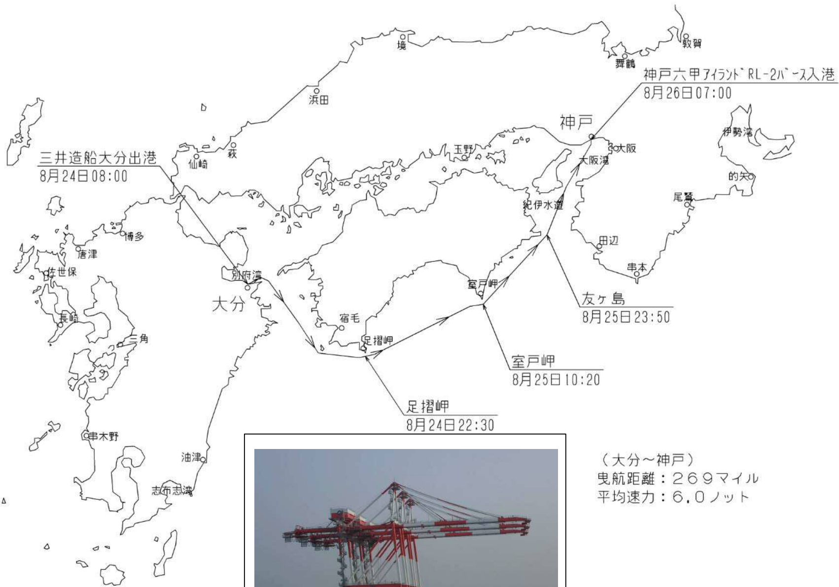
曳航経路図 (大分～神戸)
